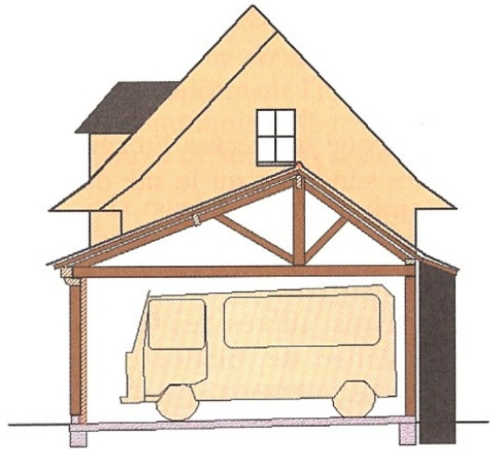
Coupe transversale des futurs garages
