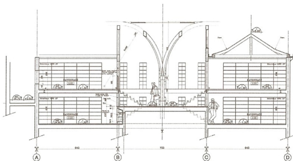
Esquisse de la coupe transversale de la future bibliothèque
